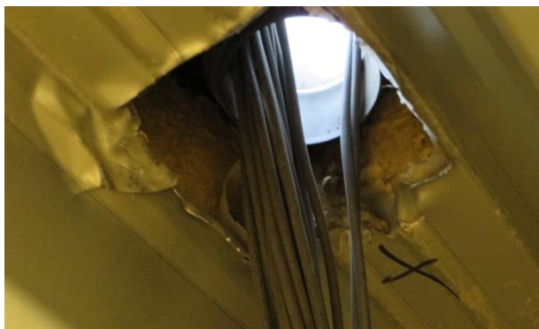
Verkeerde dakdoorvoer
